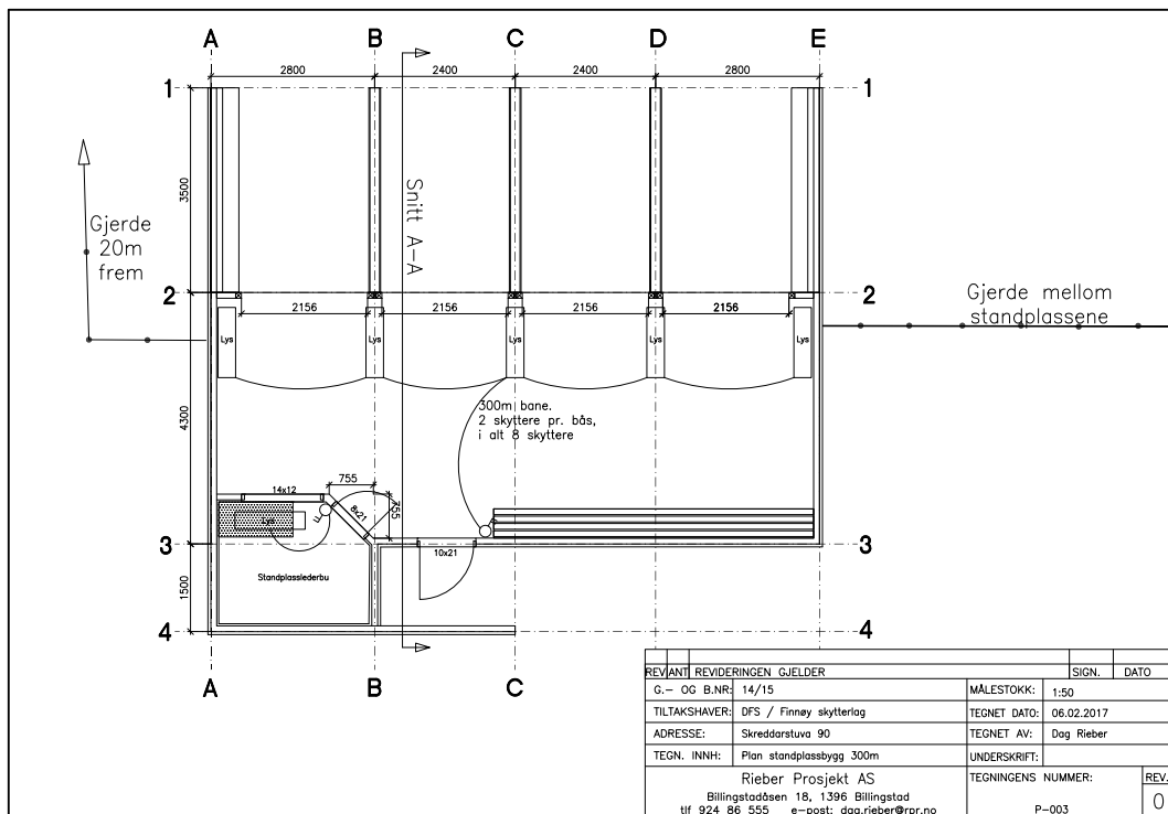
Plantegninger standplassbygg.
