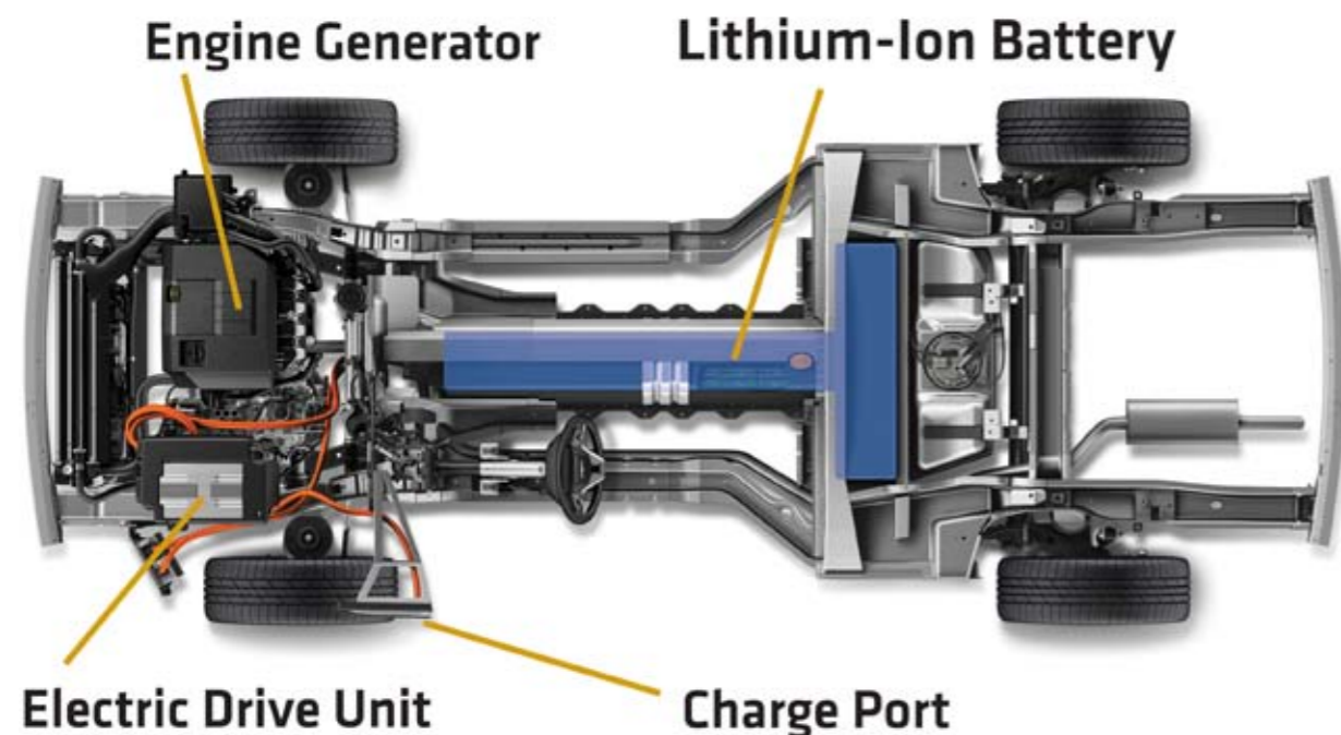
GM har bygd sine batteripakker i T-form, noe som gjør det enklere å utforme chassiset for ulike modeller. © GM Corp.
