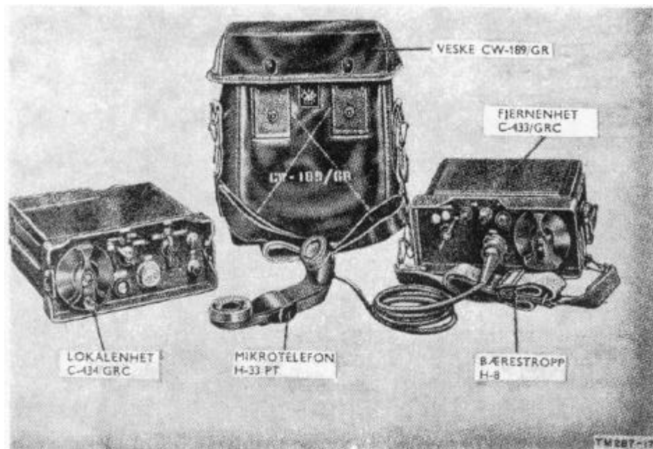
Figur 2 AN/GRA-6 fjernstyring
