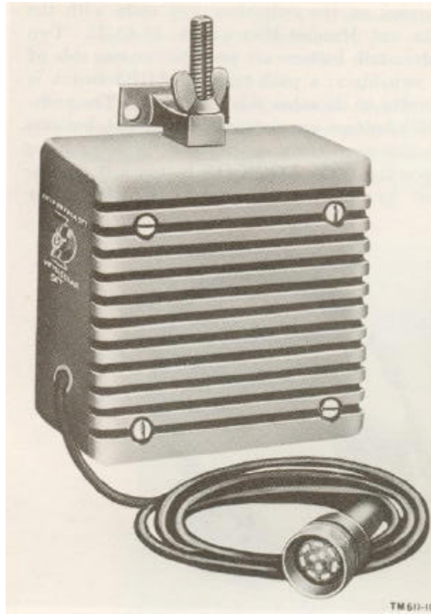
Figur 4 Høytaler LS-166
