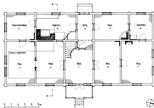
Hovedbygning på Svarstad i Sursum kommune. Plan 1. etasje. Skjematisk oppmåling (kjøpbeholdning) av Vegard Rohne i juli 2007
