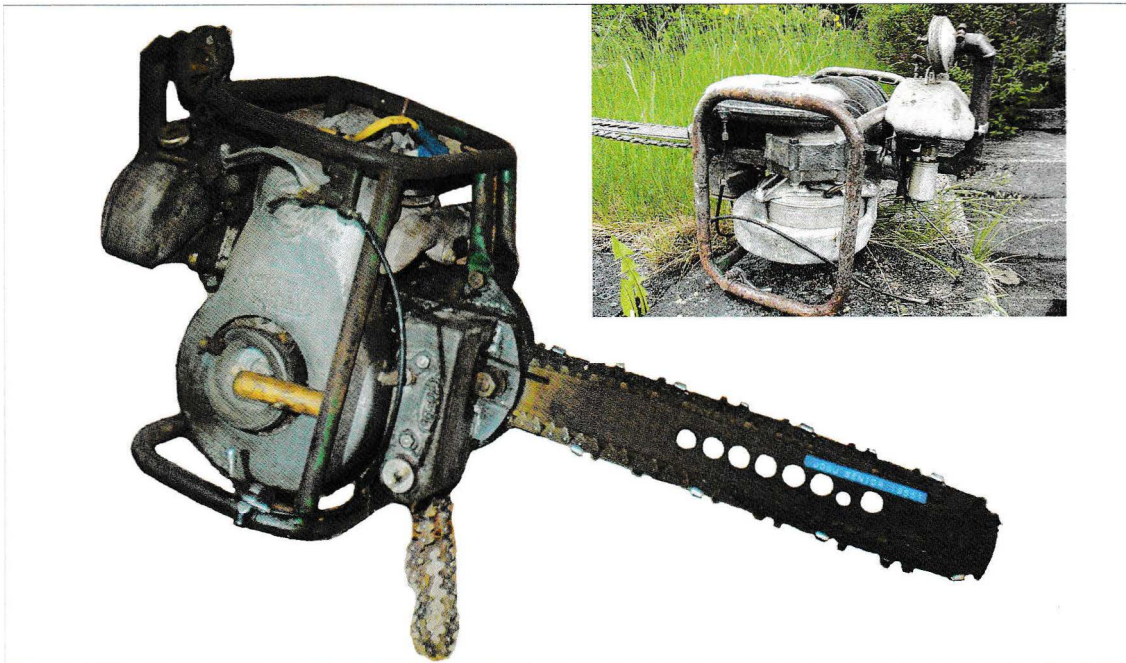
Jobu senior motorsag, øverst sees motorsagen i fellingsposisjon.
