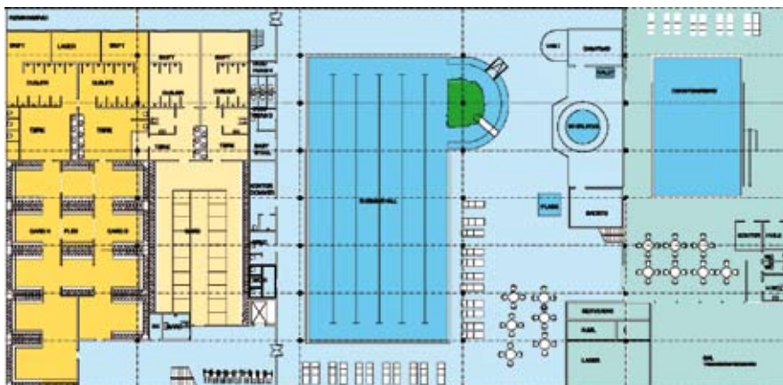
Figur 3: Arealplan for svømmehall beliggende i underetasjen mellom blokk B og C. (Kilde: Finvold Prosjekt Consult AS.)
