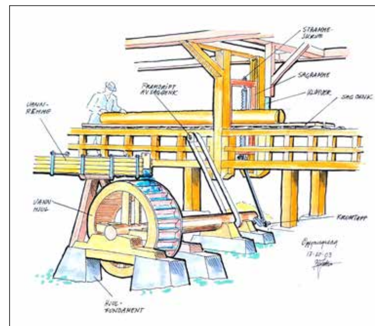
Oppgangssag, en pengemaskin noen hver kunne bygge seg. Ill.: PJS.
