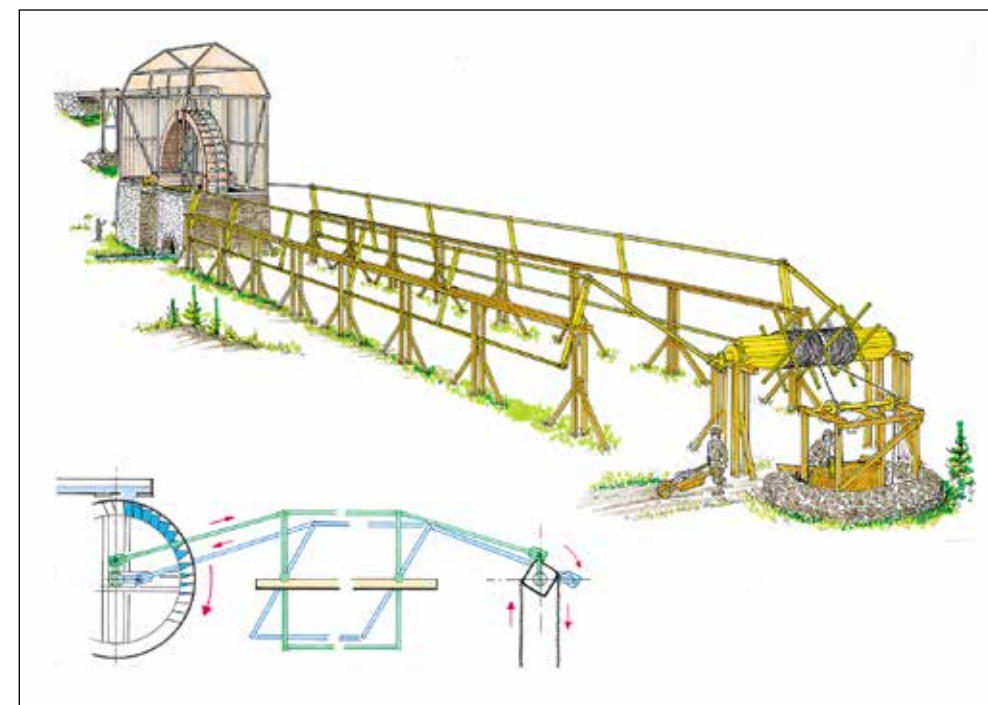
Stangkjerrat, bergverksnæringens mest kompliserte maskin. Hjulet har dobbel skovle-gang og kan således rotere begge veier. Kraften overføres til gruva via to stangfelt. PJS.
